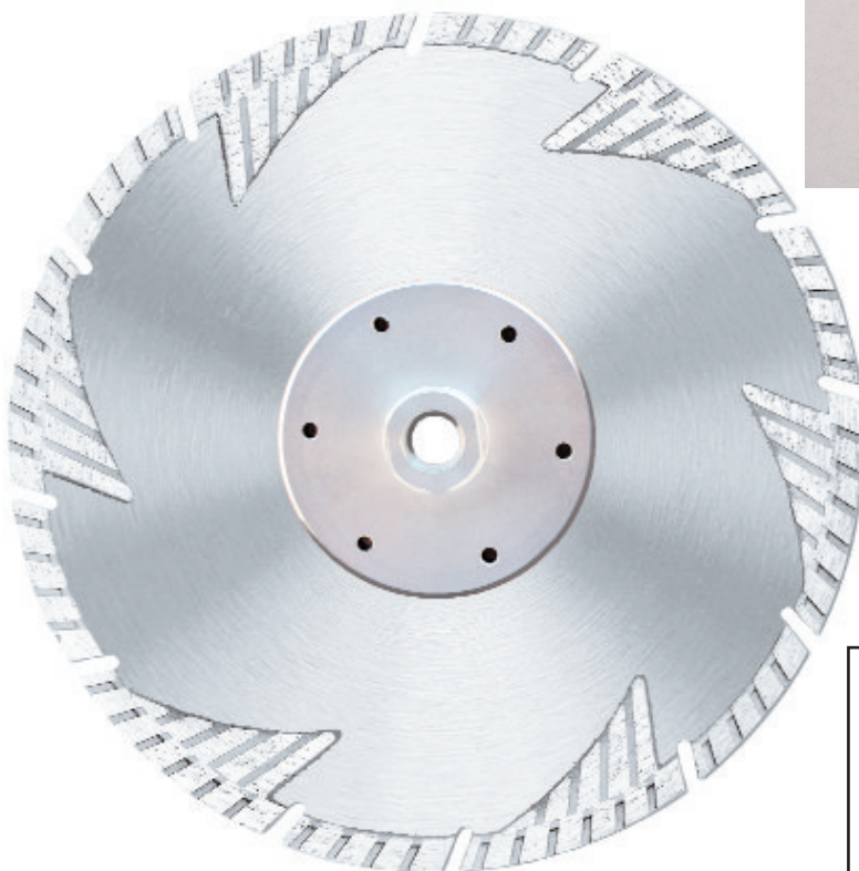
Abb. 2: mit Kern-Schutzsegmenten
